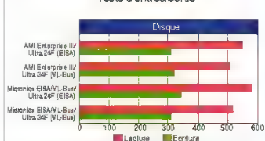
Figure 1 - Les tests disques révèlent des performances équivalentes pour les deux cartes mères en utilisation de périphérique VL-Bus. On note cependant que la carte mère Micronics EISA/VL-Bus constitue une base de conception EISA un peu plus rapide.
